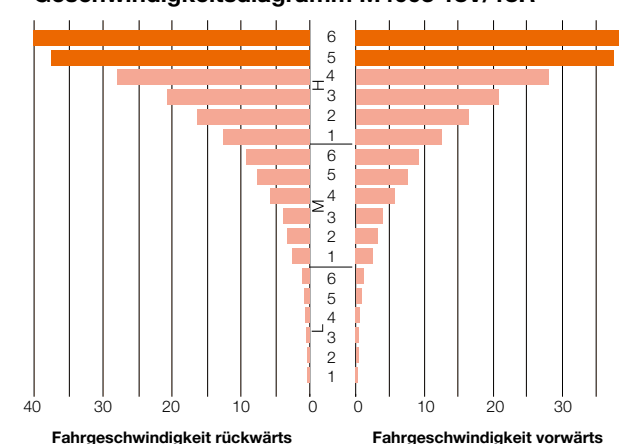
Geschwindigkeitsdiagramm M4003 18V/18R
