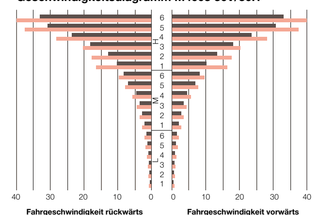
Geschwindigkeitsdiagramm M4003 36V/36R
