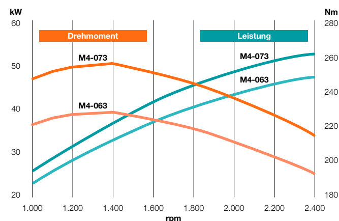
Leistung und Drehmoment
